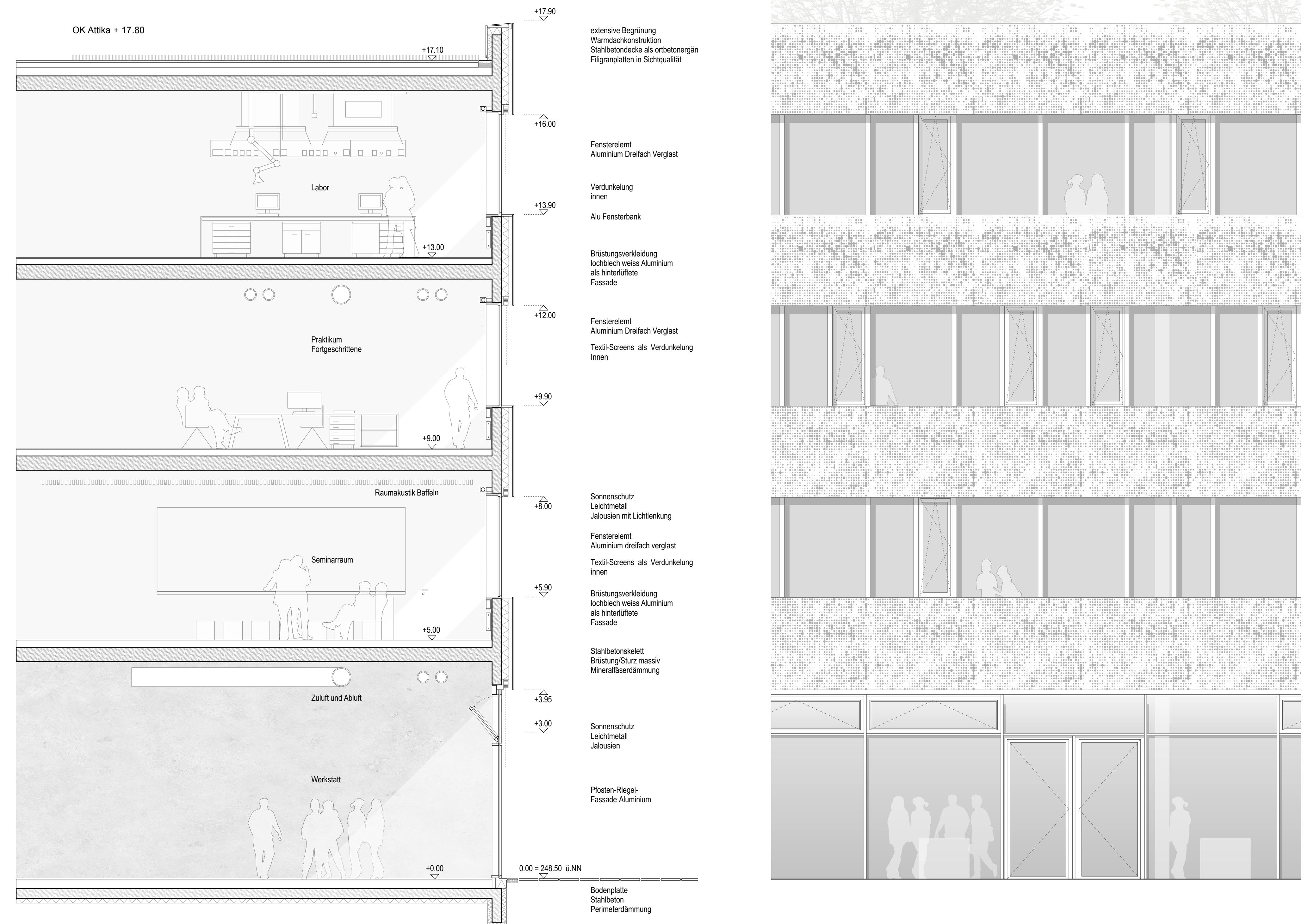
Fassadenschnitt_Teilansicht M 1_50
