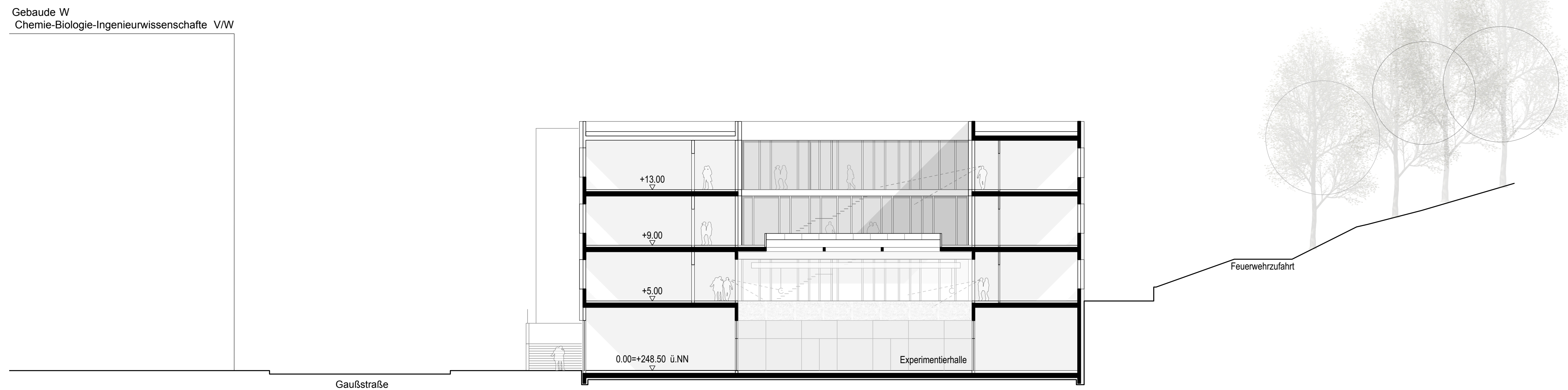
Schnitt 1-1 M 1_200
