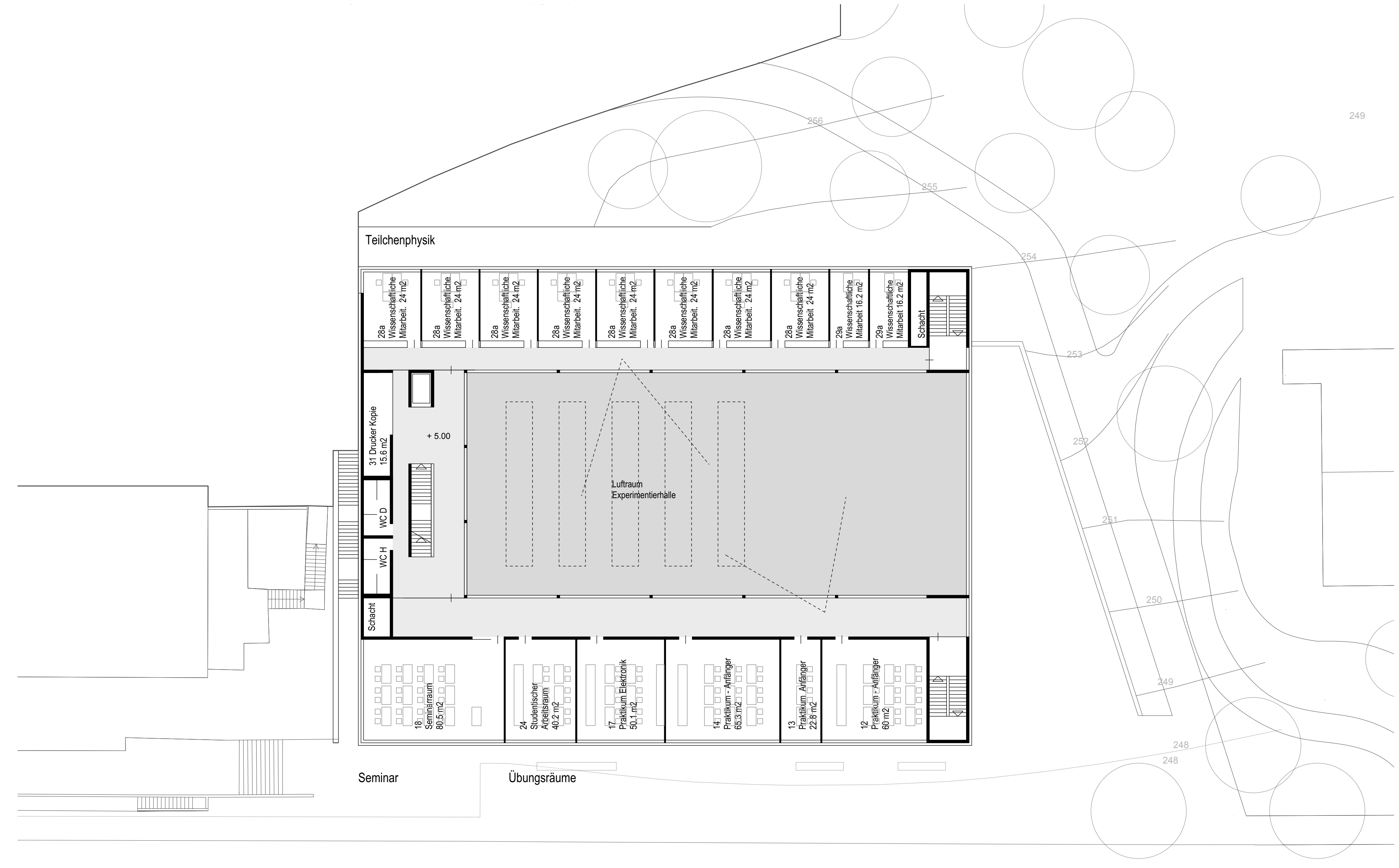
Grundriss E1 M 1_200
