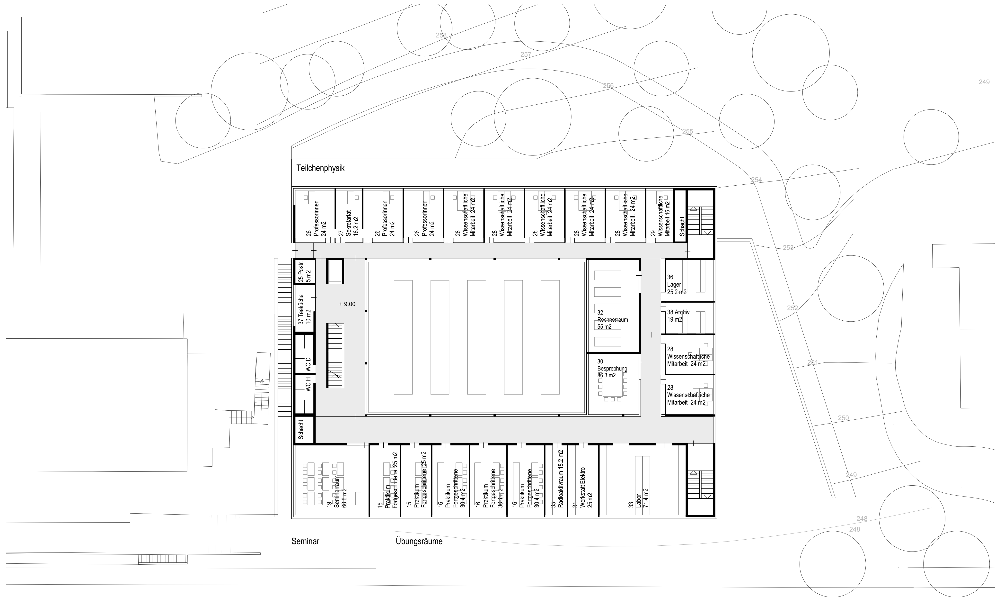
Grundriss E2 M 1_200
